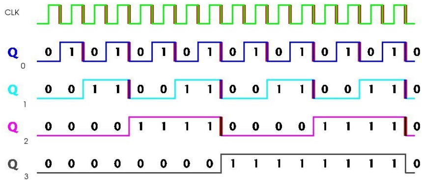
Dvojkový čítač 0...15, 0...15, ...
