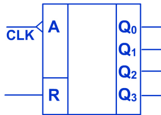
Dvojkový čítač 0...15
