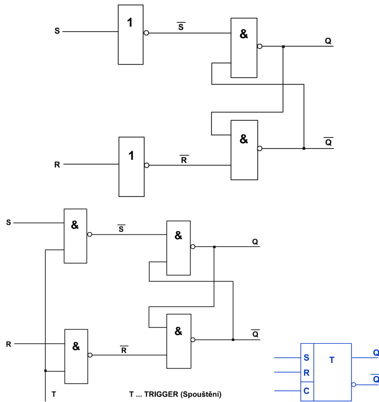
Obvod RS řízený jedničkami s časovou synchronizací.
