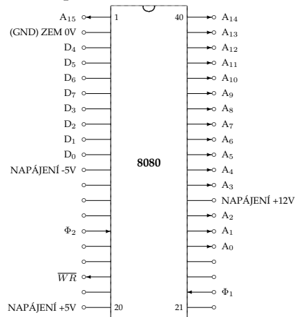
8bitový procesor
