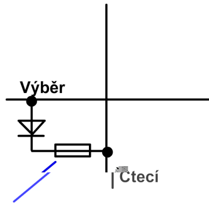
Tavná spojka NiCr
